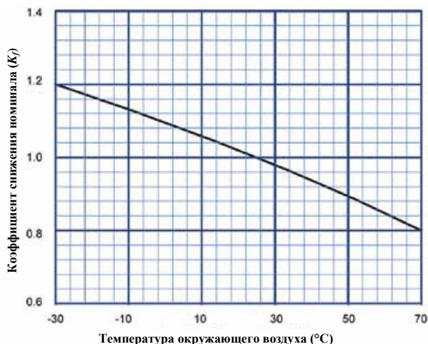
Рис. 3. График снижения номинала при аномальных температурах окружающего воздуха компании «Mersen»
