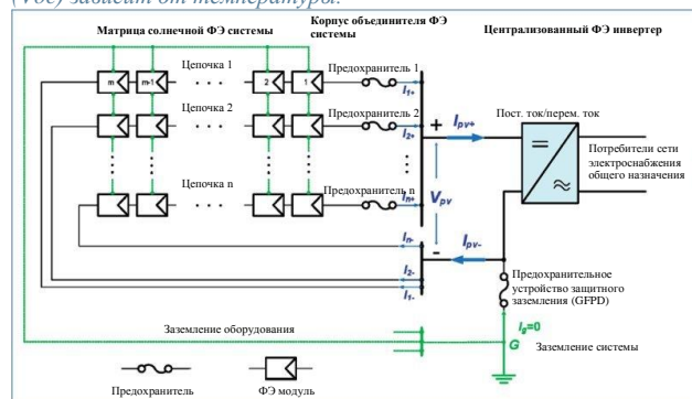
Рис. 1. Принципиальная схема включенной в сеть электроснабжения общего назначения типичной ФЭ системы при нормальных условиях
